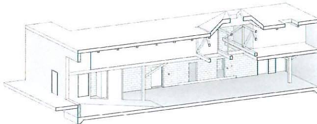
② Axo 02 - Long Section N
